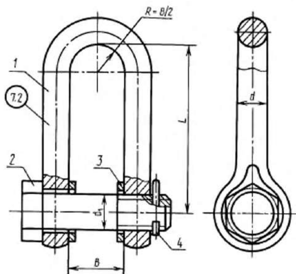
1 — скаба; 2 — болт по ГОСТ 7798 (до 48 мм) или по ГОСТ 10602 (св. 52 мм); 3 — шайба по ГОСТ 9649; 4 — шплинт по ГОСТ 397
