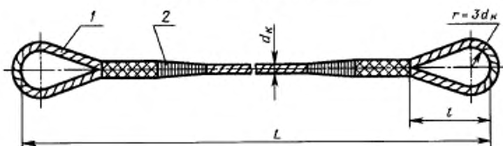
Строп с заделкой каната заплеткой
